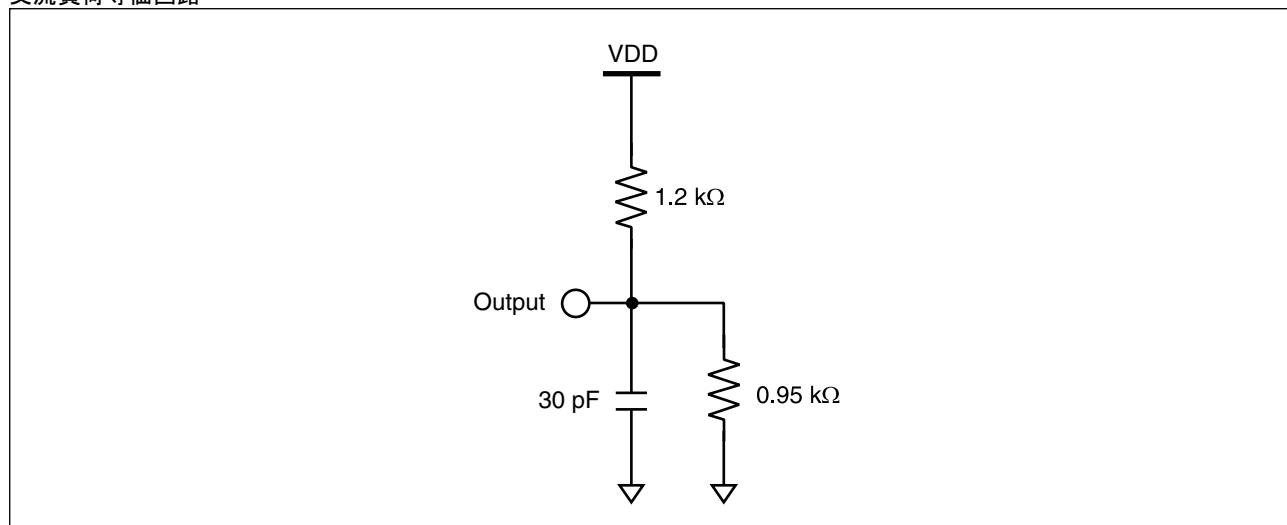
交流負荷等価回路
