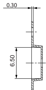
SEC.B-B
