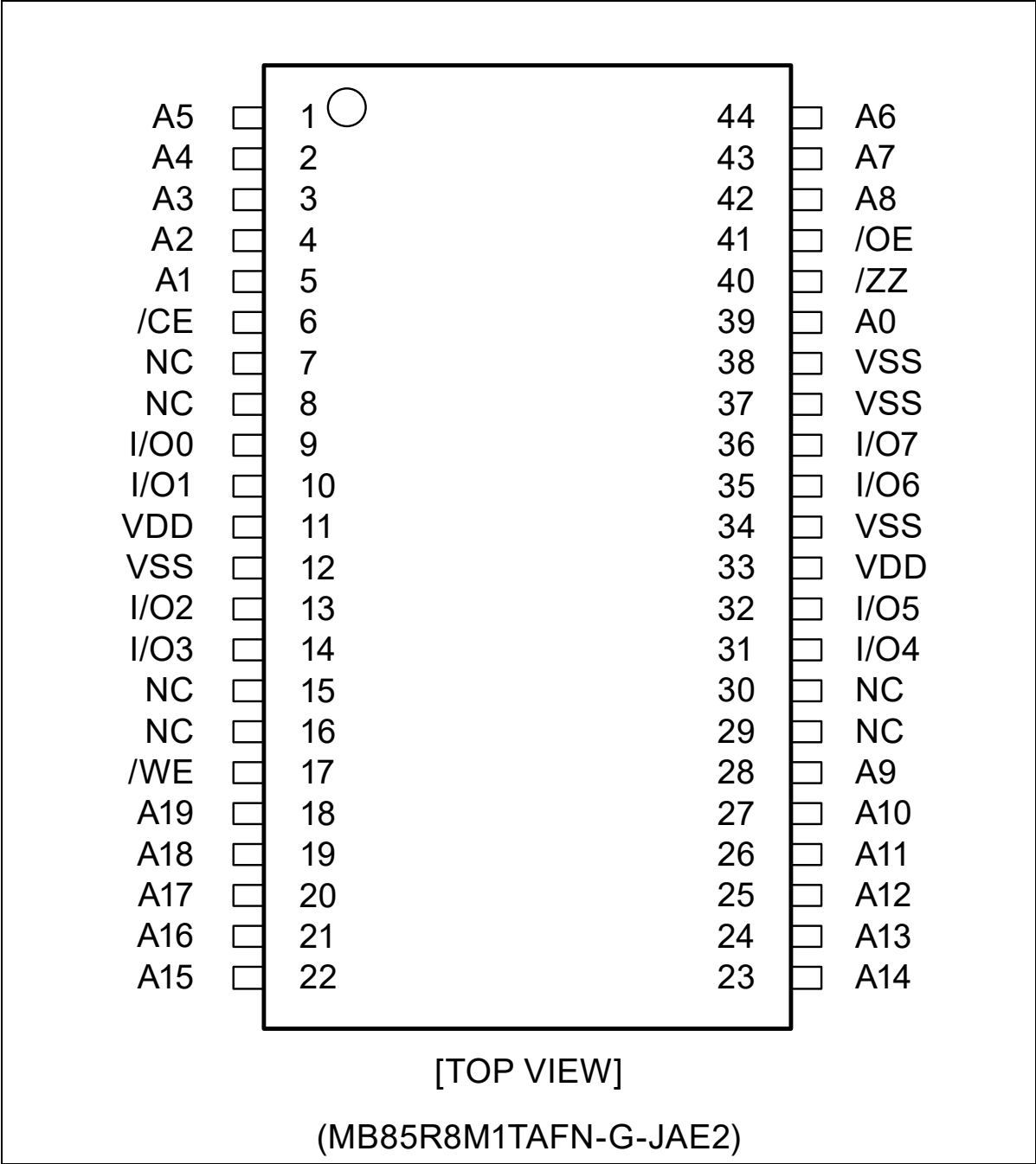
端子配列図（続き）
