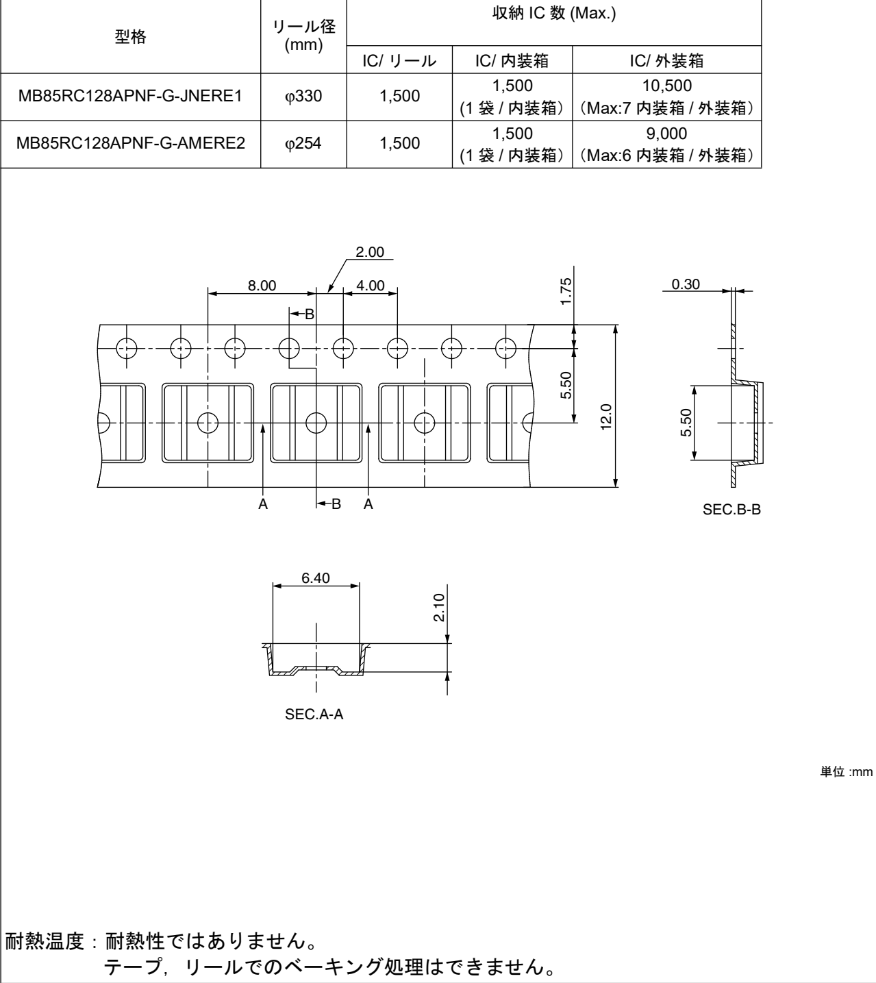
2.1 テープ寸法図 ( 模式図 )( プラスチック SOP, 8 ピン ,150mil)
