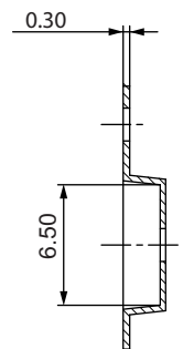
SEC.B-B
