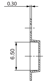
SEC.B-B
