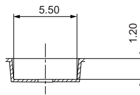
SEC.A-A
