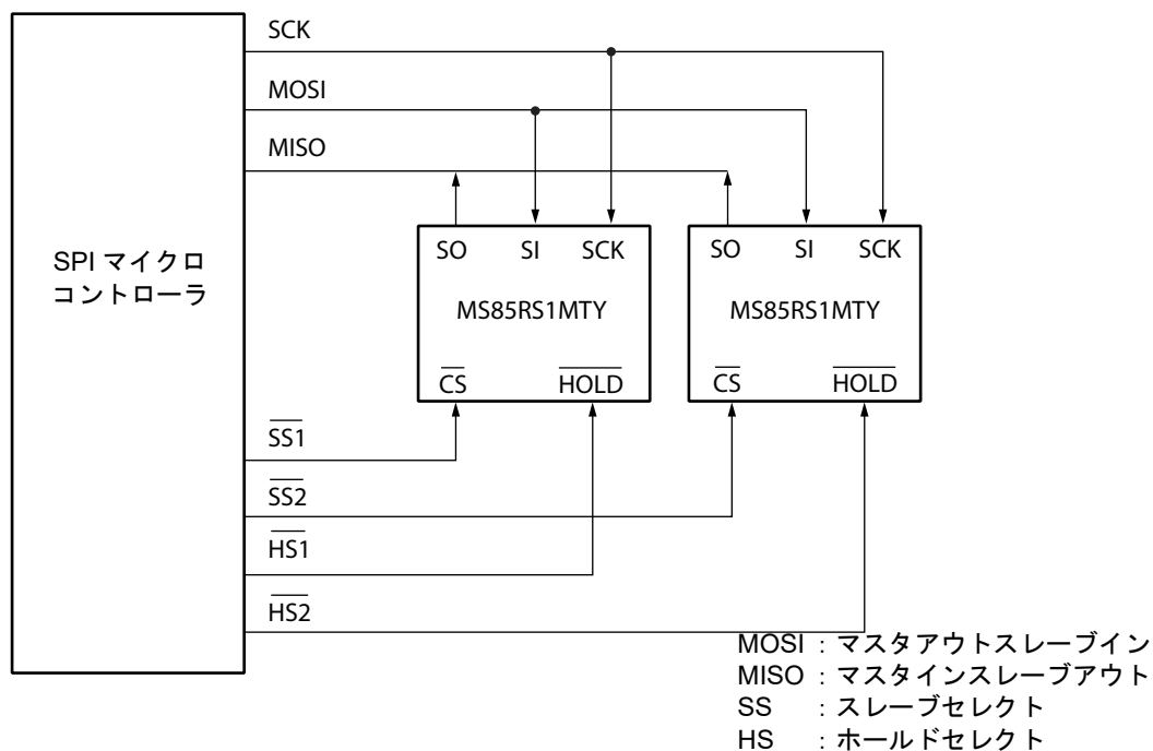
SPI ポートがある場合のシステム構成図
